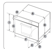
Dimensions requises pour l'installation
