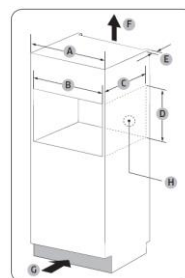
Meuble encastré (mm)
